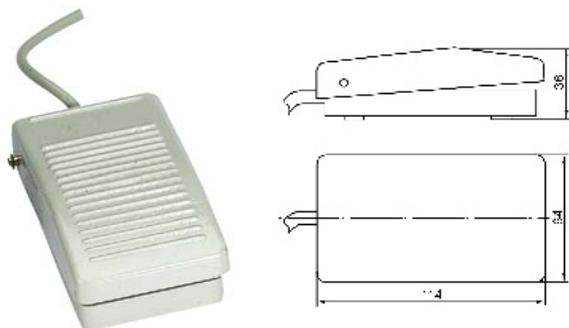
LLJFS1-3(铝壳Aluminum cover)
